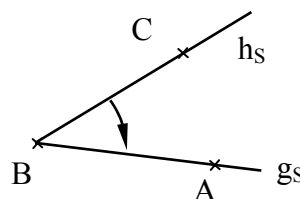
negativer orientierter Winkel
