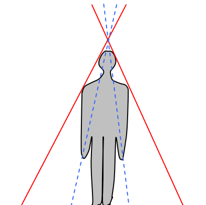
Winkeldrittung
