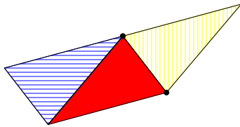
beim Parkettieren
