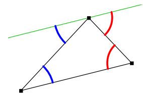
durch Winkelsätze an Parallelen
