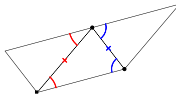
über Punktspiegelungen
